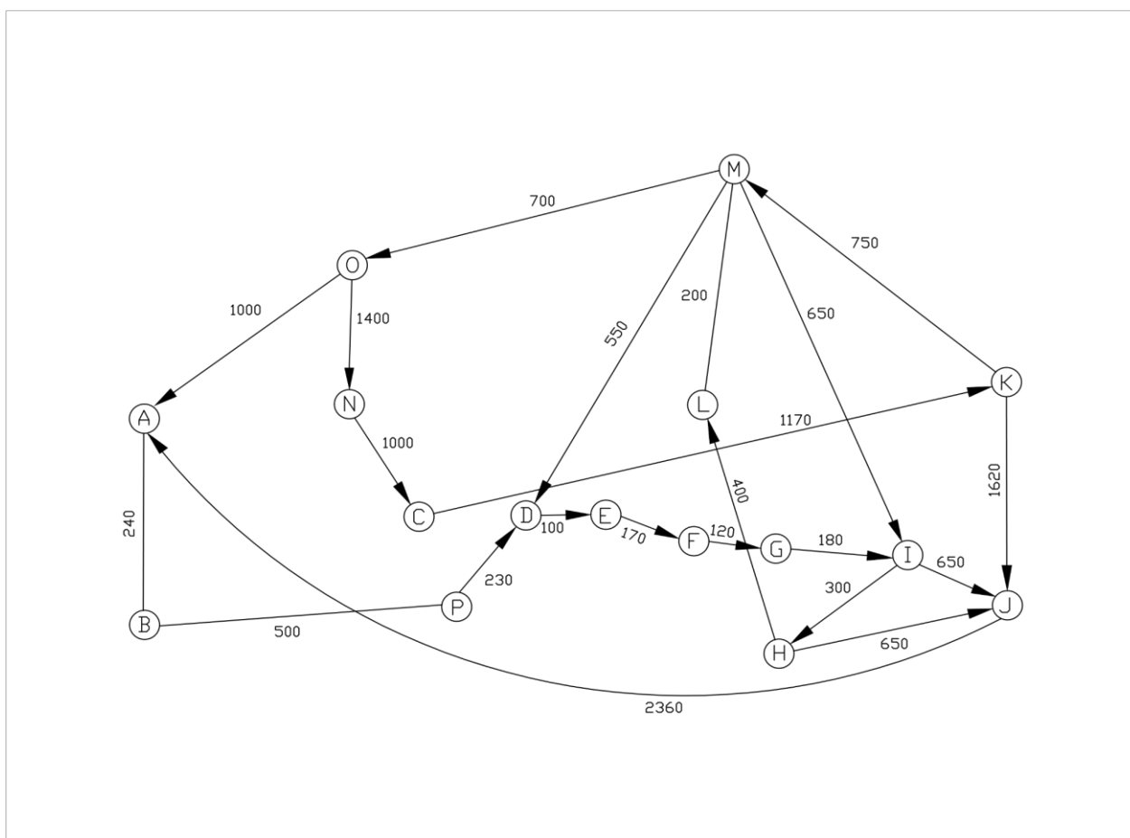
Slika 6. Rješenje TSP algoritmom umetanja najbližeg
