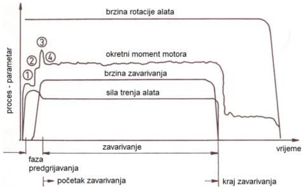
Slika 8. Dijagram promjene parametara kod FSW zavarivanja[11]:
