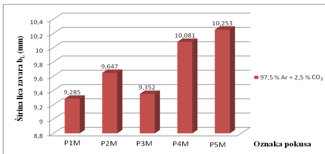
Slika 60. Histogram širine lica zavara, 97,5 % Ar + 2,5 % CO 2 .
