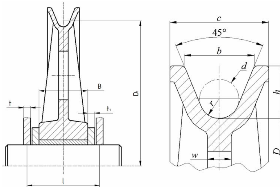
Slika 4.2 Dimenzije i profil žlijeba užnice
