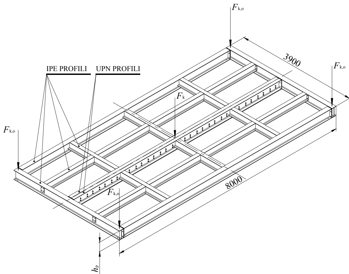
Slika 3.1 Nosiva konstrukcija
