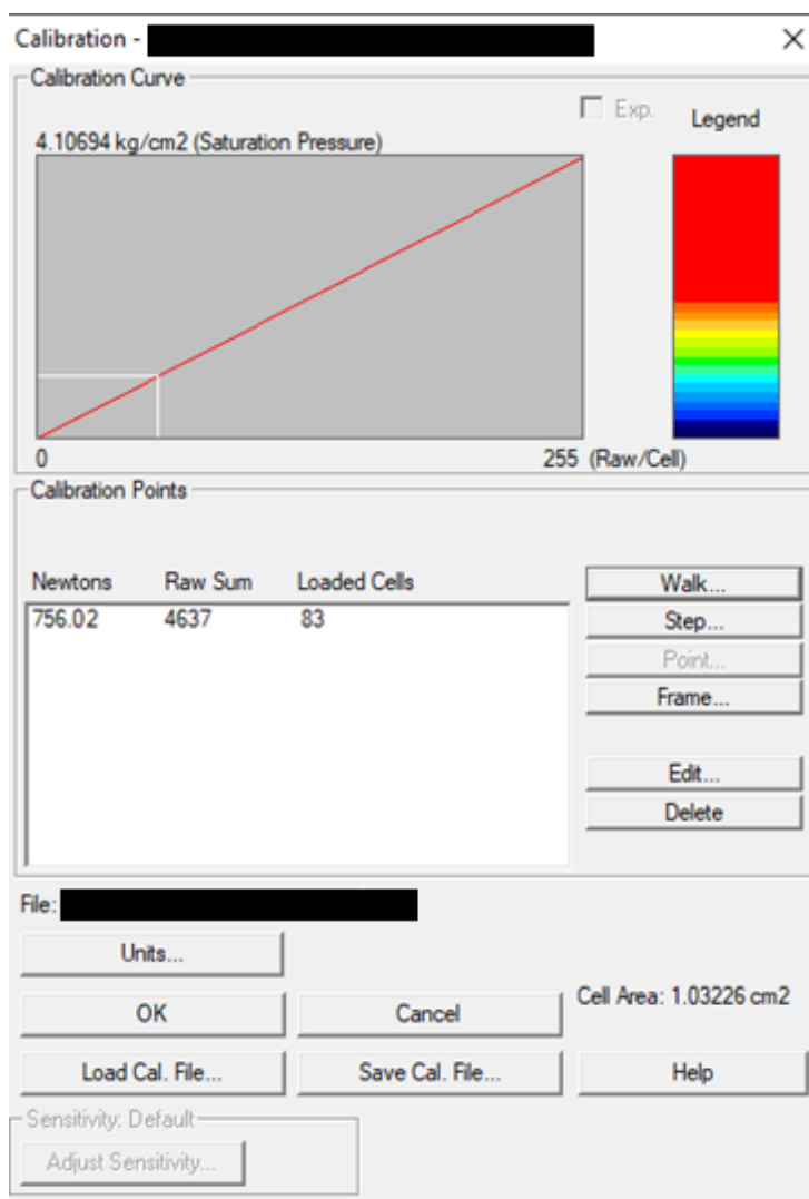
Slika 27. Kalibracija platforme
