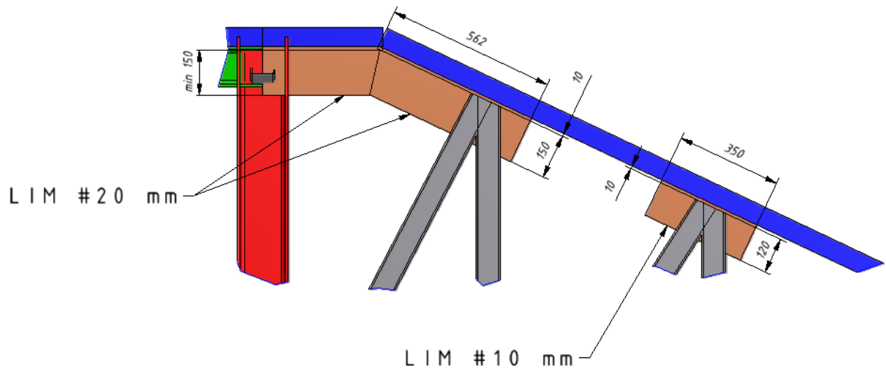
Slika 4.4 Ojačanja u gornjem pojasu vodilica U-160, kombinacijom limova
