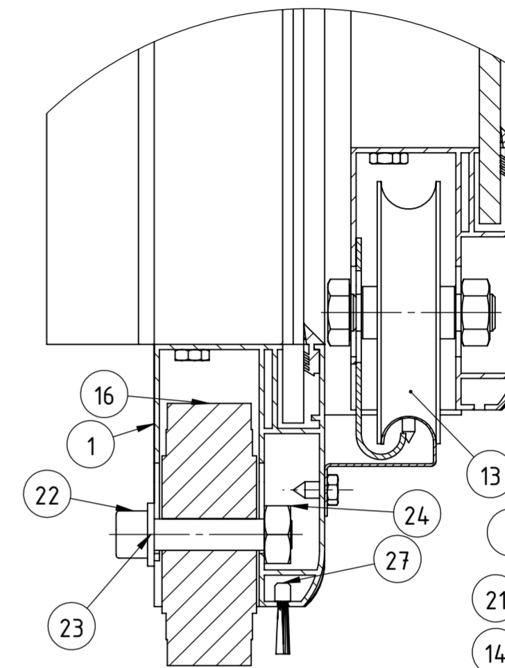
DETALJ D (1 : 2)
