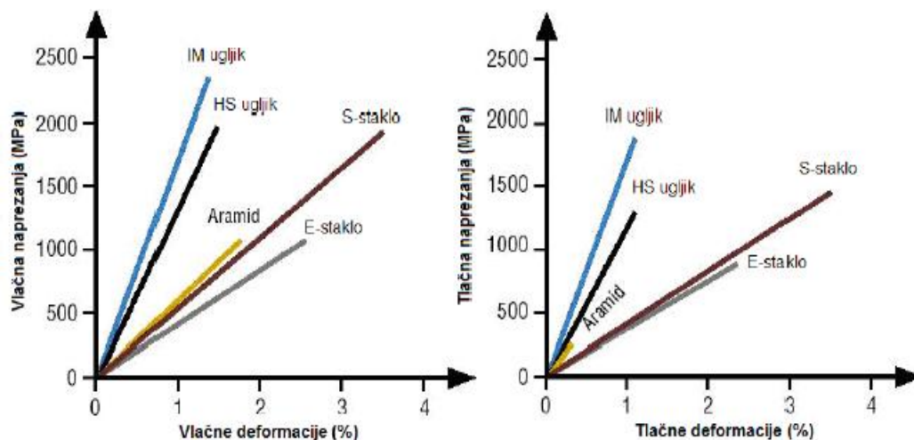
Dijagram 2.2 odnosi napreznja i deformacija različitih vrsta vlakana
