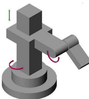
Slika 2.3. Kvazicilindrična struktura robota
