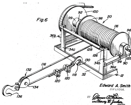
Slika 6. Patent US3322398A [4]
