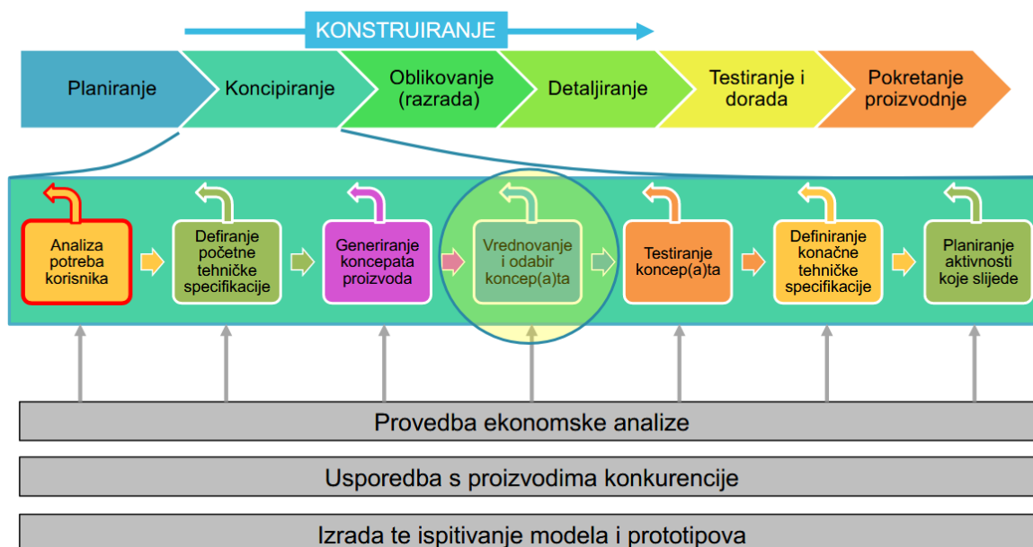
Slika 4. Faze konstruiranja [15]
