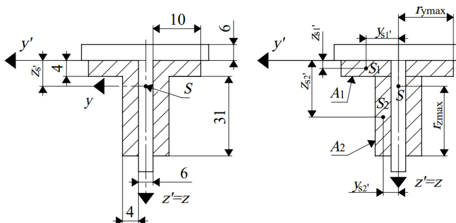
Slika 31. Dimenzije prvog zavara
