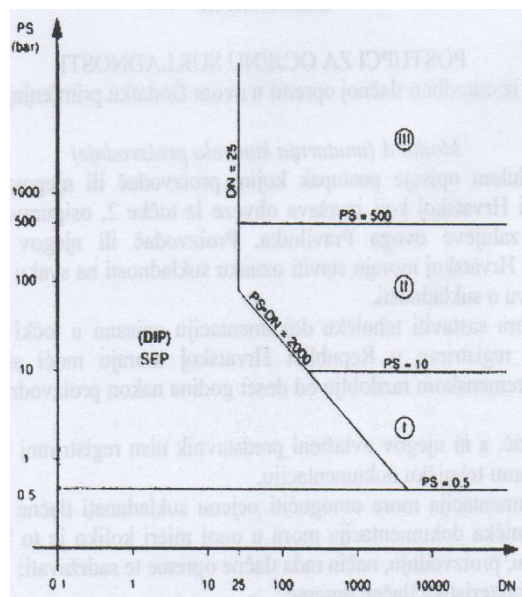
Dijagram 8. Cjevovodi za kapljevinske grupe 1
