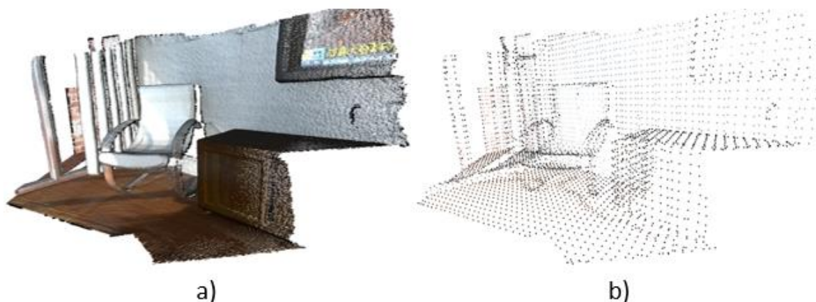
Slika 2.11 a) Učitani oblak točaka u Open3D [21], b) Obradjeni oblak točaka unutar Open3D-a[21]
