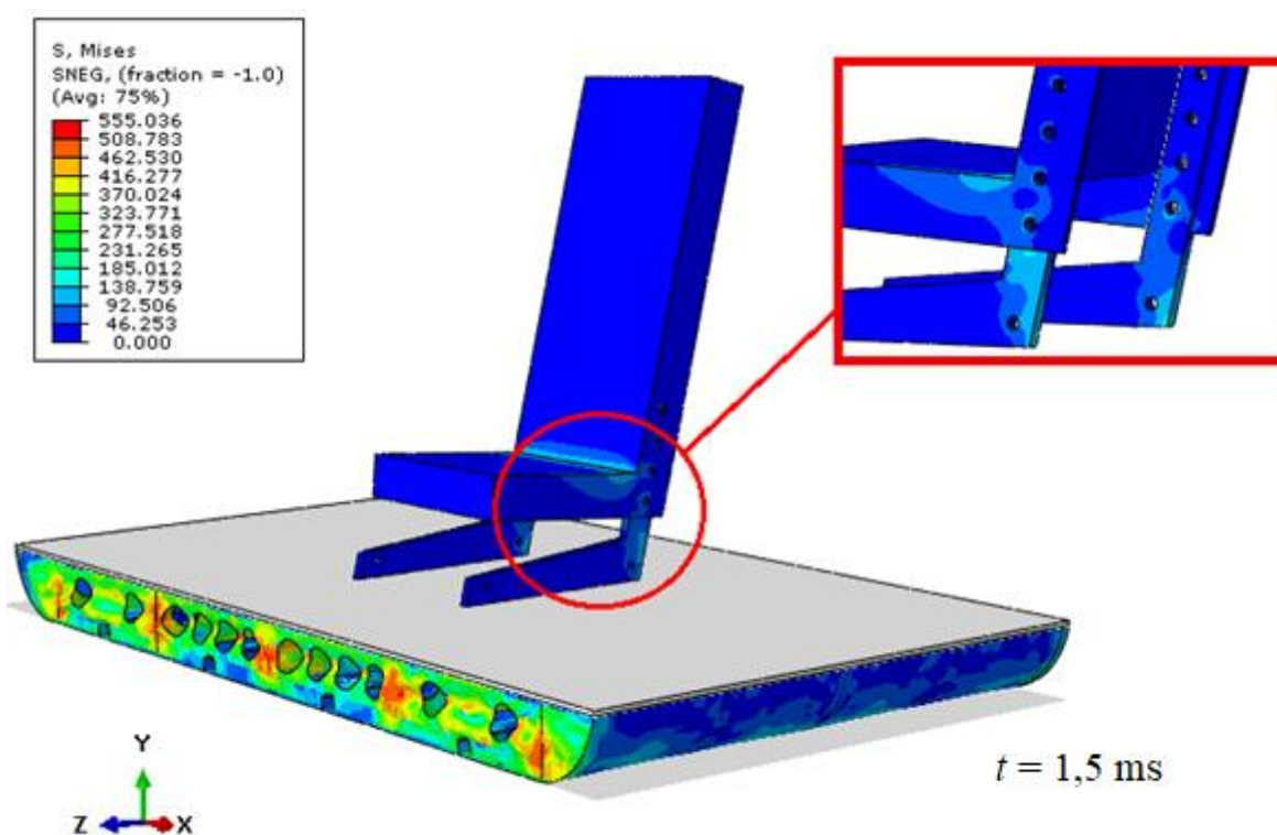
Slika 25. Ekvivalentno von Mises napreznja aluminijskog sjedala u trenutku 1,5 ms [MPa]
