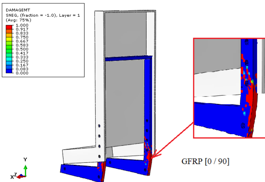
Slika 49. Prikaz oštećenja [-] koje nastaju na sjedalu GFRP kompozitnog materijala za DAMAGEMT [0/90]
