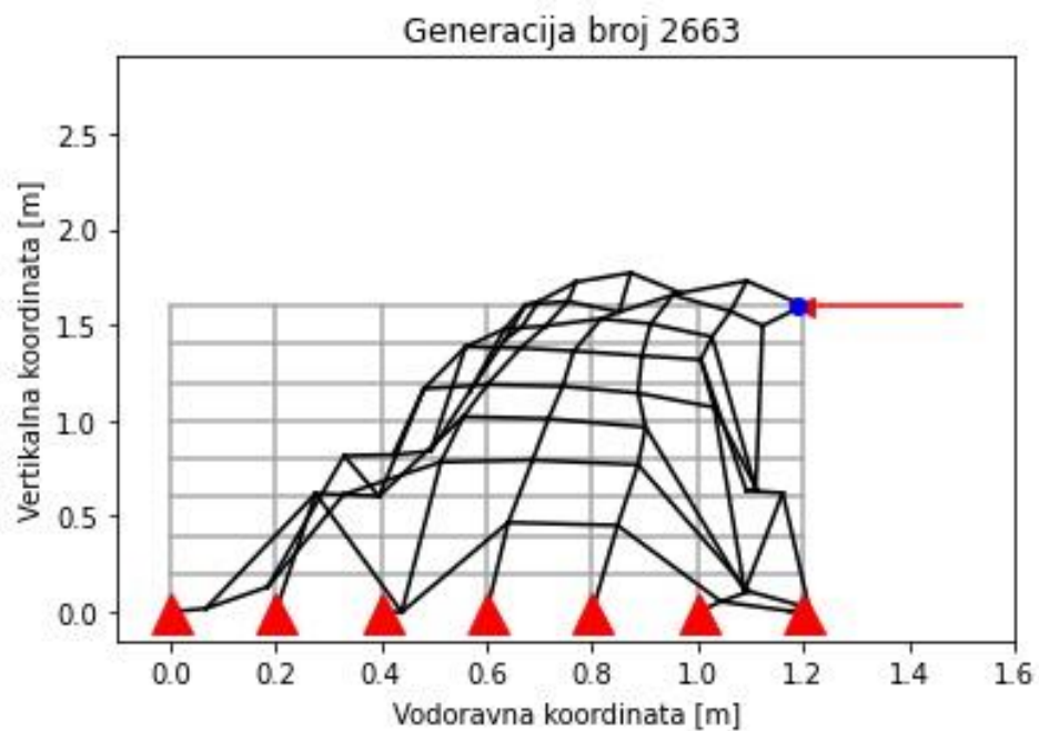
Slika 33. Prvi pokus evolucije koso opterećene konstrukcije
