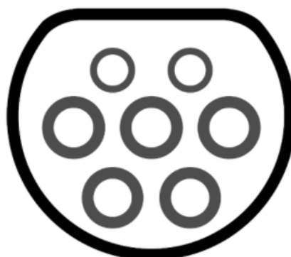
Slika 9. Priključak-TIP 2 [14]
