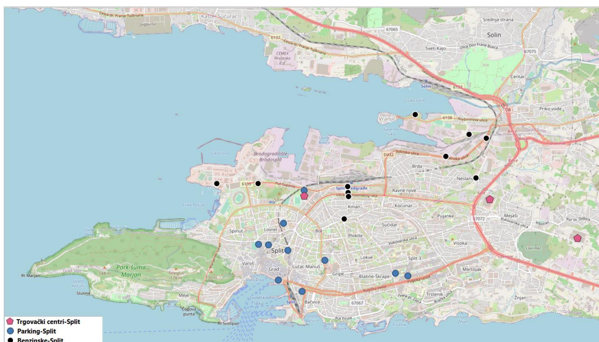
Slika 33. Potencijalne lokacije punionica električnih vozila u gradu Splitu
