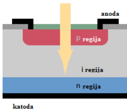
Slika 18. PIN fotodiode [17]
