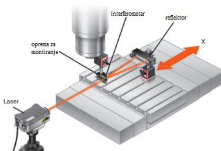
Slika 15. Skica sustava za mjerenje pravocrtnosti pomoću interferometra [14]
