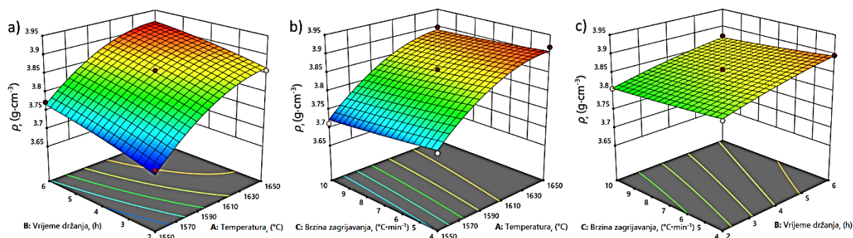
Slika 8.16 Prikaz utjecaja procesnih varijabli: a) temperatura sinteriranja (A), b) vrijeme držanja (B), c) brzina zagrijavanja (C) na postignutu gustoću sinteriranih uzoraka pomoću 3D-odzivnih površina.
