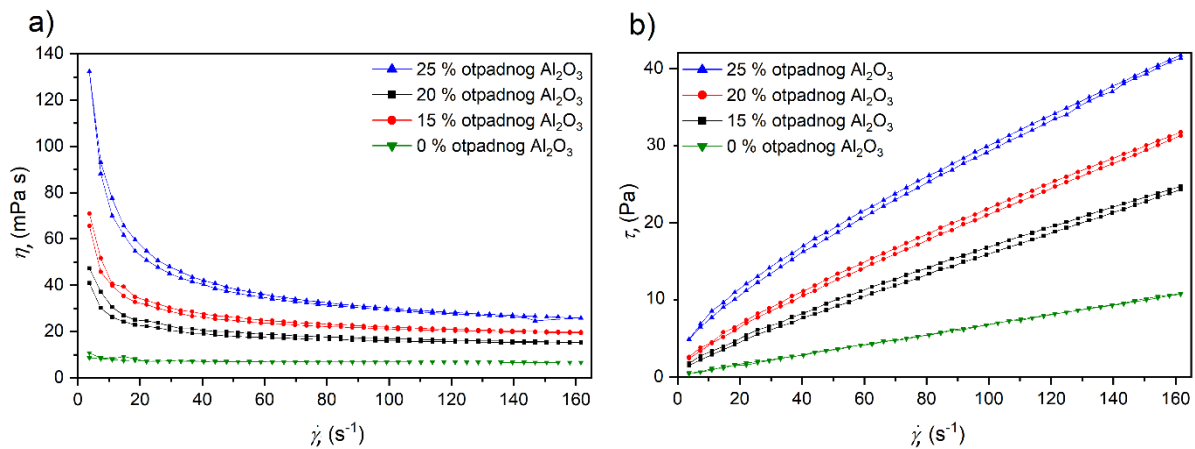
Slika 8.7 Keramičke suspenzije (70 % masenog udjela) s različitim udjelima otpadnoga praha a) ovisnost prividne viskoznosti o smičnoj brzini, b) ovisnost smičnog napreznja o smičnoj brzini.
