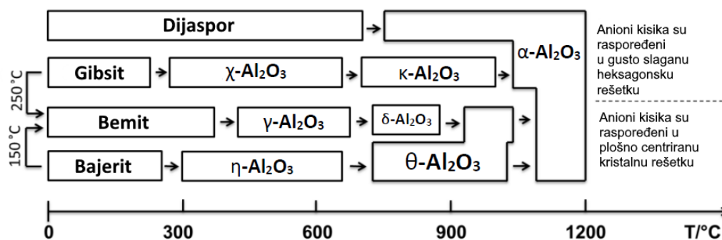
Slika 3.2 Prijelazi kristalnih modifikacija aluminijeva oksida [53].
