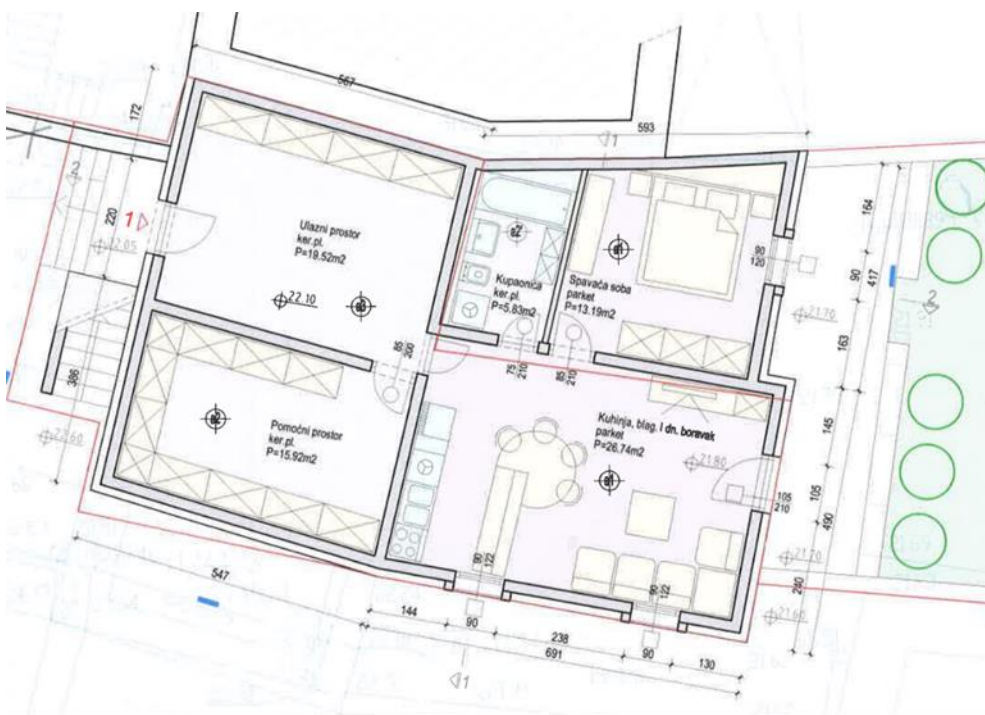
Slika 8. Tlocrt prizemlja
