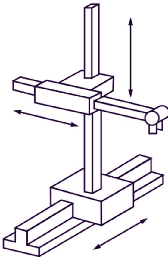
Slika 13. Kartezijev robot [10]
