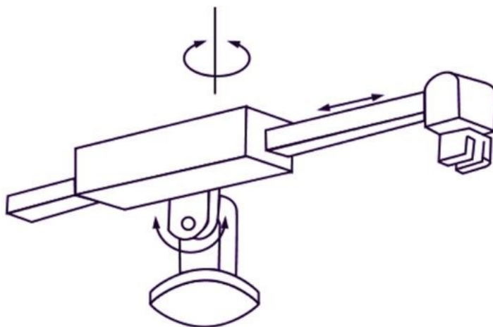
Slika 16. Polarni robot [13]
