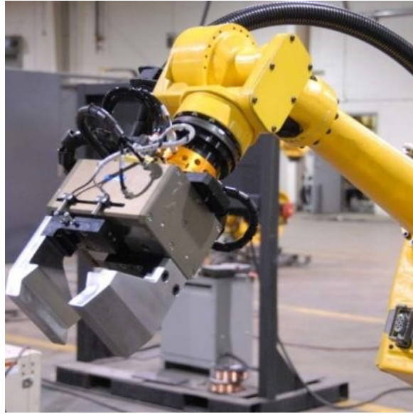
Slika 22. Hidraulička hvataljka [19]
