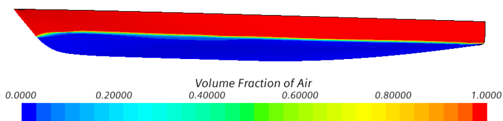
Slika 38. Slobodna površina po vanjskom dijelu trupa katamarana s razmakom H/L = 0,3 pri Fr = 0,5
