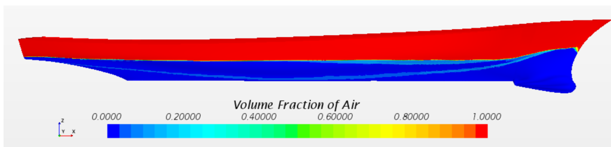
Slika 26. Slobodna površina uzduž golog trupa za finu mrežu
