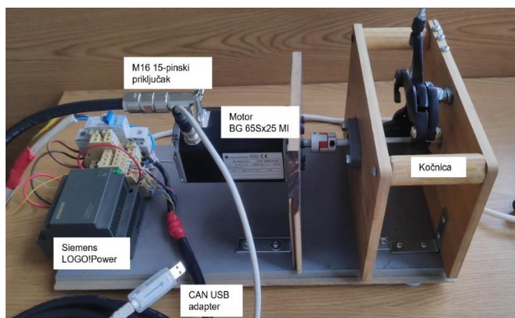
Slika 35. Eksperimentalni postav
