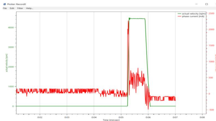
Slika 37. Integrirani osciloskop
