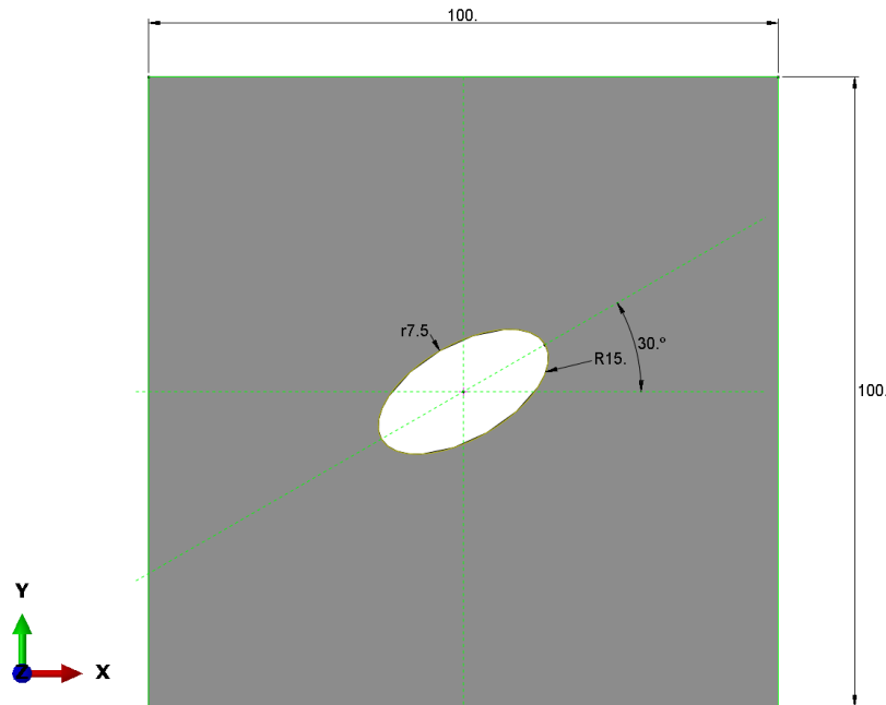
Slika 17 Elipsa zakrenuta za 30^\circ s odnosom stranica a/b = 2 i a/H = 0,15
