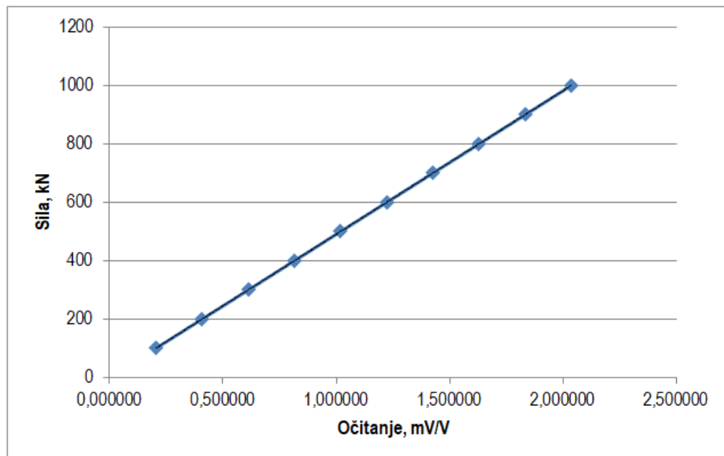
Slika 29. Inverzna interpolacija vrijednosti umjeravanja utega do 1000N
