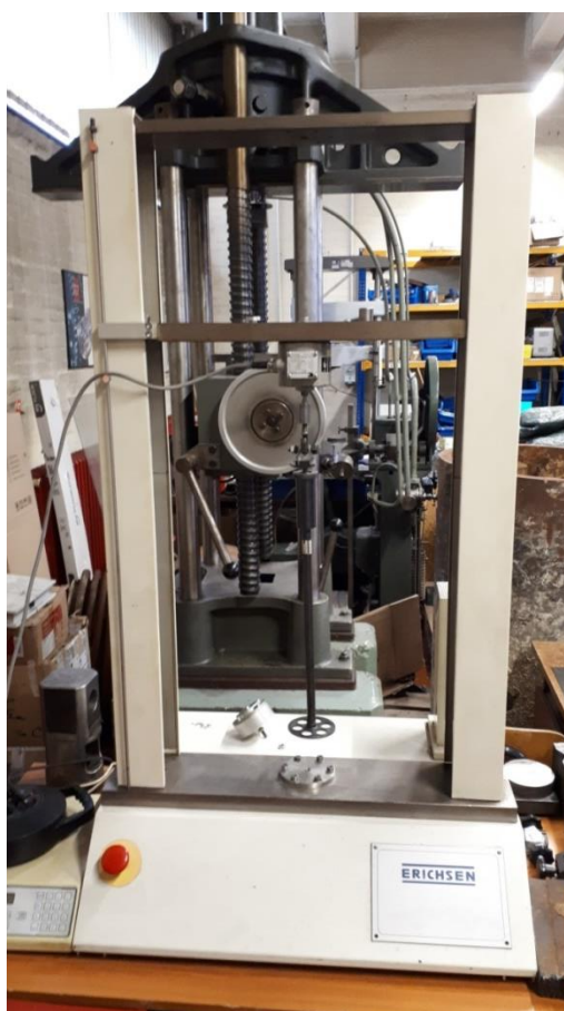
Slika 23. Kidalica Laboratorija za mehanička ispitivanja Fakulteta strojarstva i brodogradnje
