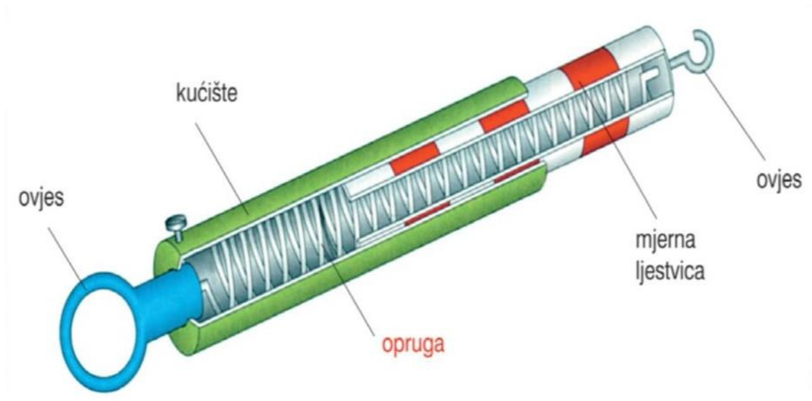
Slika 7. Dinamometar [16]
