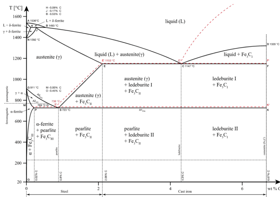
Slika 17. \text{Fe}-\text{Fe}_3\text{C} dijagram [18]
