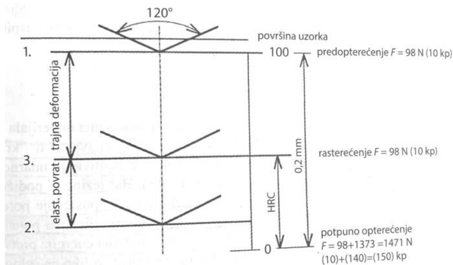
Slika 3. Rockwell-ova metoda [2]
