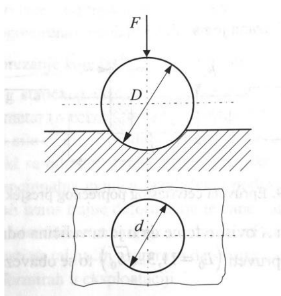
Slika 1. Brinell-ova metoda [2]
