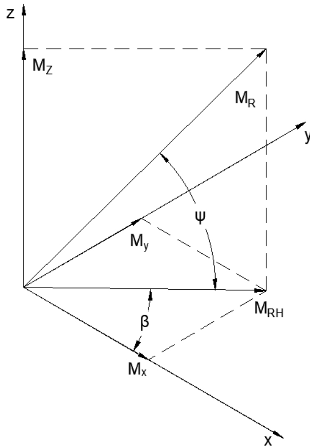
Slika 48. Prostorni prikaz određivanja rezultatnog momenta M_R
