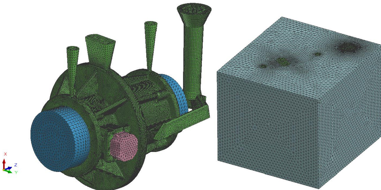
Slika 70. Elementarni dijelovi odljevka, jezgre te uljavnog sustava
