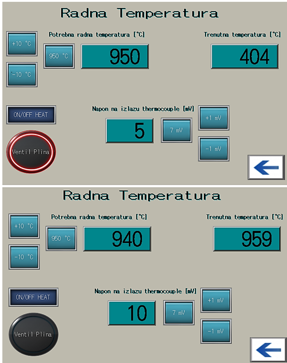
Slika 48. Radna temperatura-grafičko sučelje
