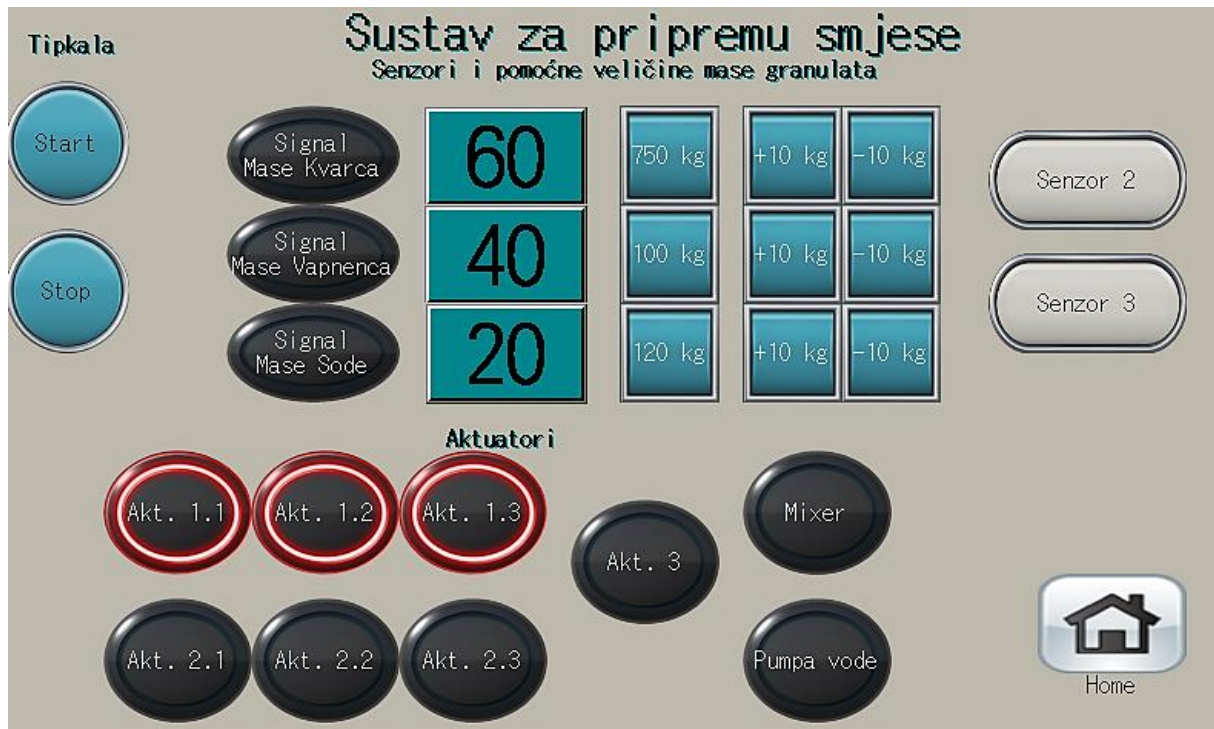
Slika 44. Grafičko sučelje sustava pripreme smjese (završetak ciklusa i početak novog)
