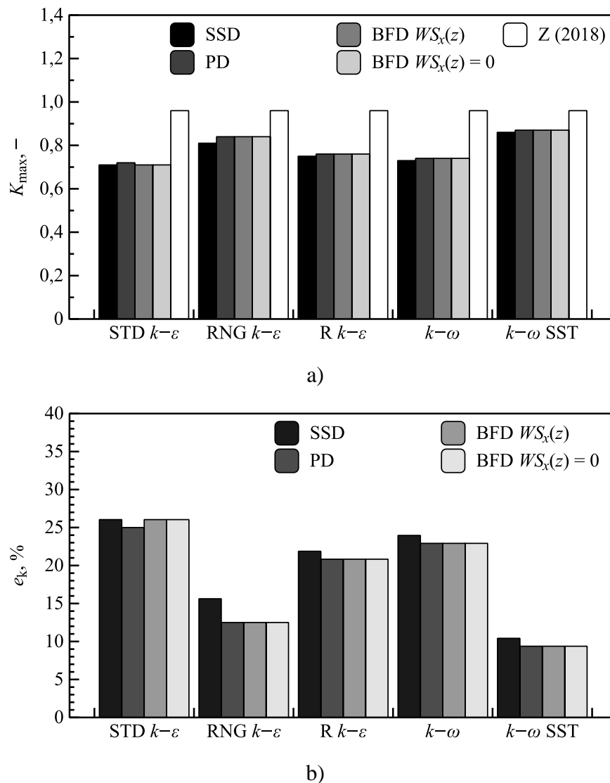
Slika 62. a) Maksimalne vrijednosti prirasta osrednjene brzine K_{\max} u usporedbi s eksperimentalnim vrijednostima [162], te b) srednje pogreške prirasta osrednjene brzine \epsilon_k dobivene računalnim simulacijama strujanja inženjerskog AGS-a oko uzdignute zgrade primjenom modela u kojima strujanja uzrokuju smična sila (SSD), sila gradijenta tlaka (PD) i dodatna masena sila (BFD WS_x(z) – s njenom primjenom i BFD WS_x(z) = 0 – bez njene primjene) promjenjiva po visini. Računalne simulacije provedene su koristeći standardni k-\varepsilon , RNG k-\varepsilon , realizable k-\varepsilon , Wilcoxov k-\omega i Menterov k-\omega SST model turbulencije.
