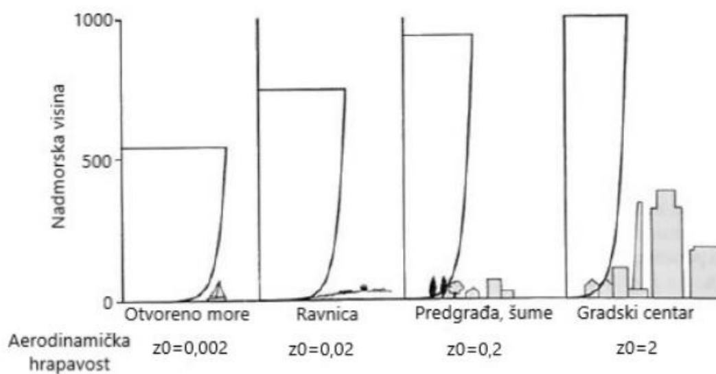
Slika 44. Aerodinamička hrapavost [23]
