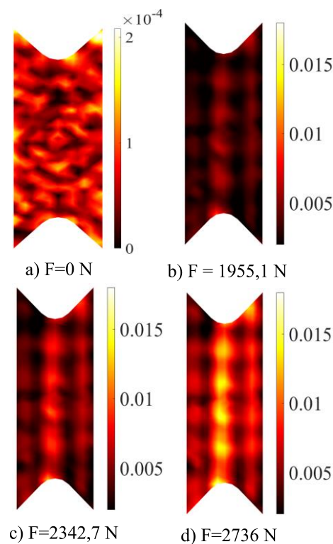
Slika 33. Polja najvećih glavnih deformacija u linearnom području mehaničkog odziva materijala monotonog ispitivanja izračunata pomoću Correli 3.0 algoritma.
