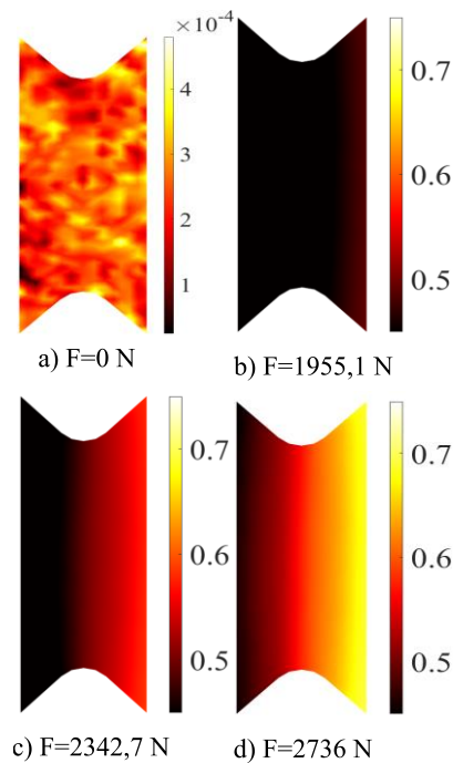
Slika 28. Polja pomaka u x -smjeru u linearnom području mehaničkog odziva materijala izmjerena pomoću Correli 3.0 algoritma za monotono ispitivanje.
