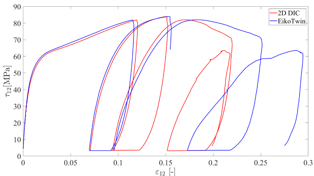
Slika 25. Usporedni dijagram deformacija - naprezanje za monotono ispitivanje.
