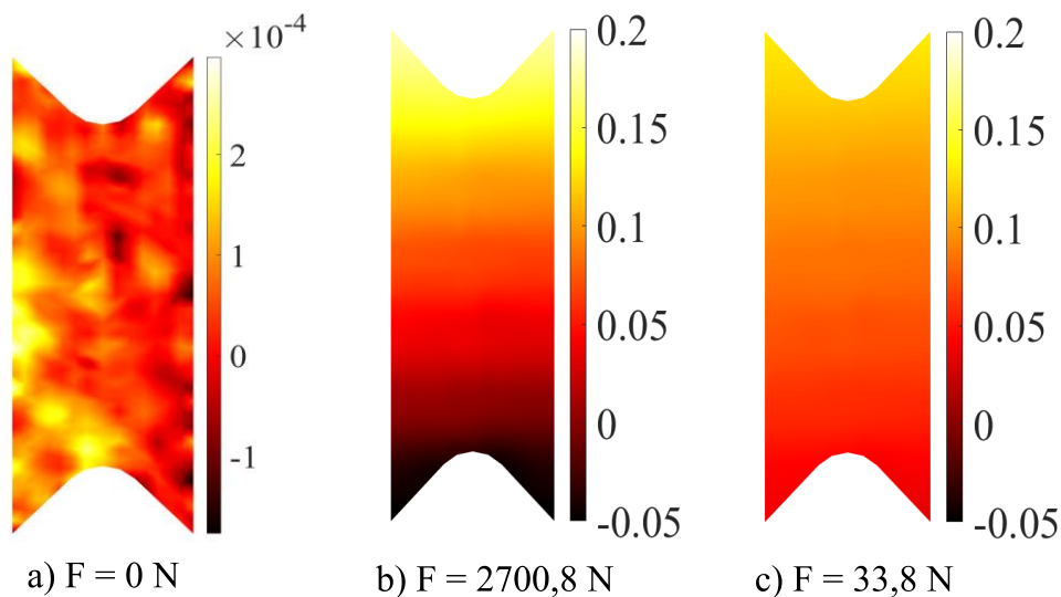
Slika 66. Polja pomaka u y -smjeru izmjerena pomoću Correli 3.0 algoritma za prvi ciklus cikličkog ispitivanja.
