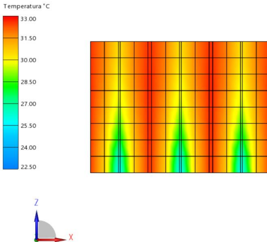
Slika 40. Temperatura prednje plohe „stack-a“ na završetku simulacije
