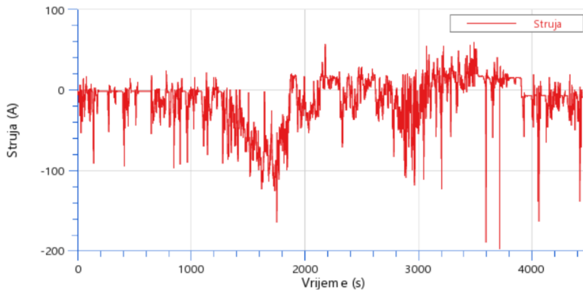
Slika 34. Struja u bateriji pri stvarnom ciklusu vožnje
