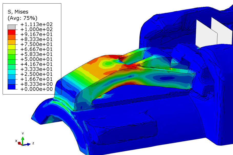
Slika 68. Raspodjela ekvivalentnog naprezanja prema von Misesu ( \text{N/mm}^2 ) na deformiranom obliku kopče za zaključavanje (svojstva materijala dobivena pomoću eksperimentalnog ispitivanja)
