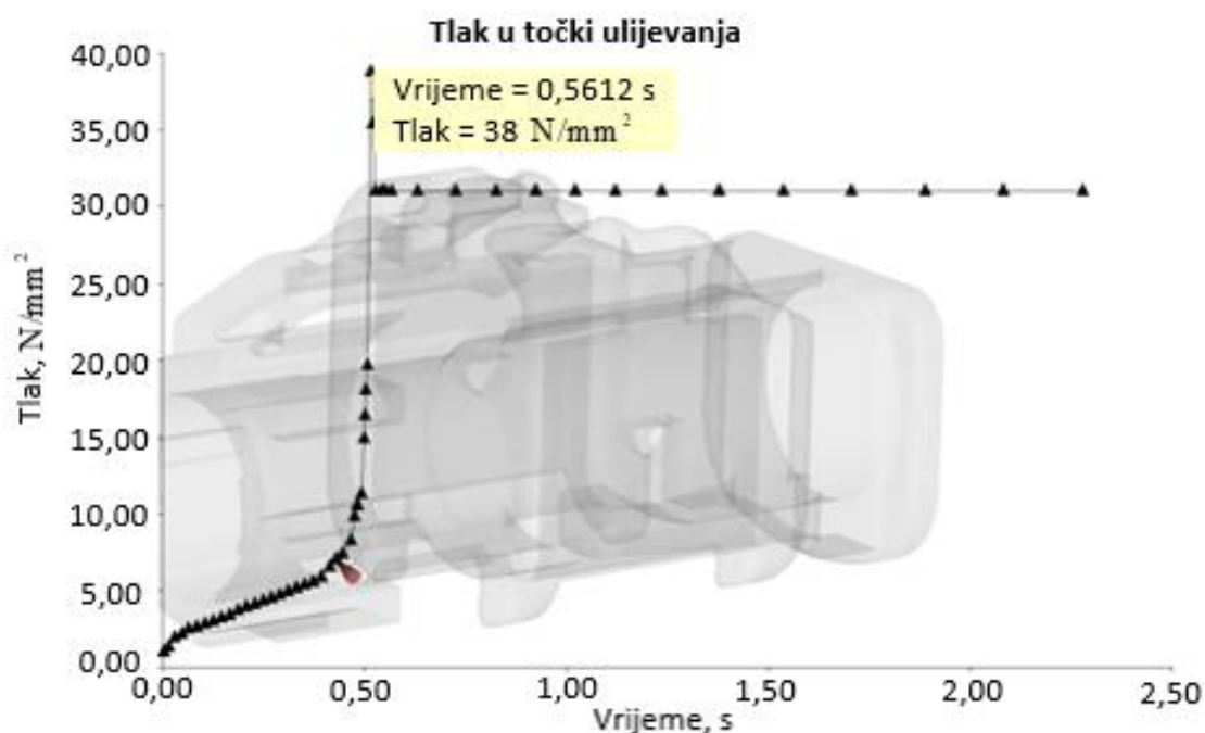
Slika 5. Promjena tlaka za vrijeme popunjavanja alata
