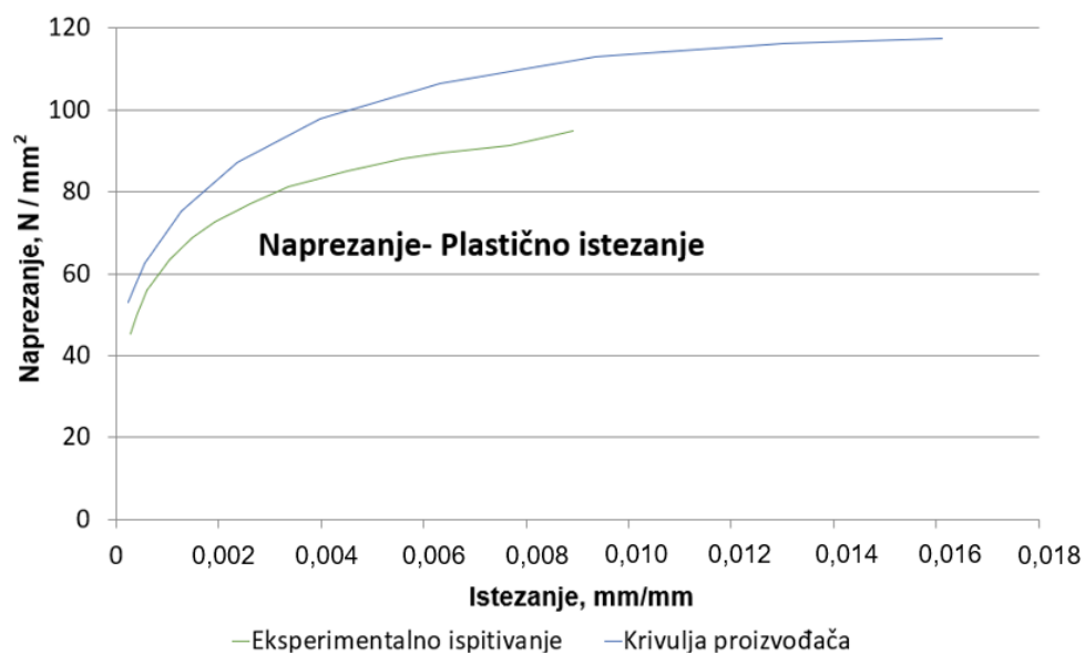
Slika 25. Dijagram naprezanje – plastična deformacija za Pocan B3225
