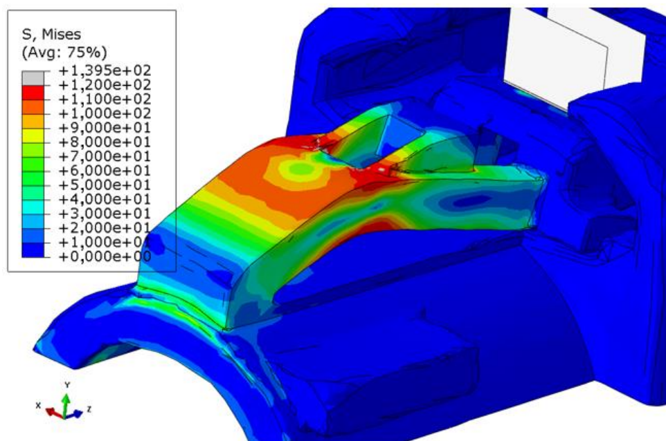
Slika 65. Raspodjela ekvivalentnog napreznja prema von Misesu (N/mm 2 ) na deformiranom obliku kopče za zaključavanje (svojstva materijala dobivena od proizvođača materijala)
