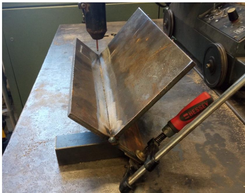
Slika 34. Priprema kutnog spoja
