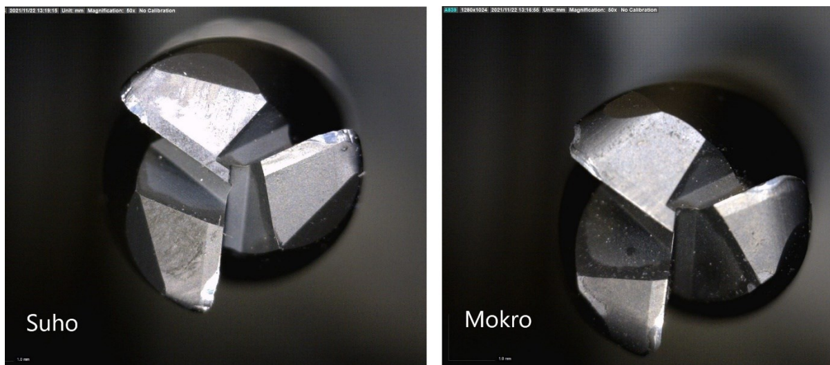
Slika 69 Prikaz trošenja stražnje površine glodala s radijusom pod mikroskopom
