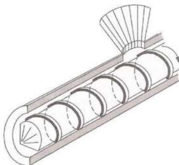
Slika 3. Jednopužni ekstruder [4]
