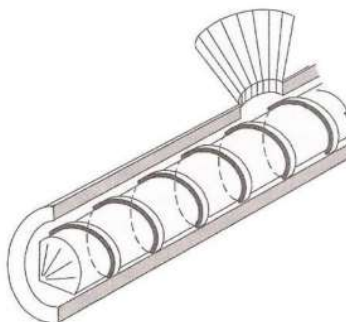
Slika 3. Jednapužni ekstruder [4]
