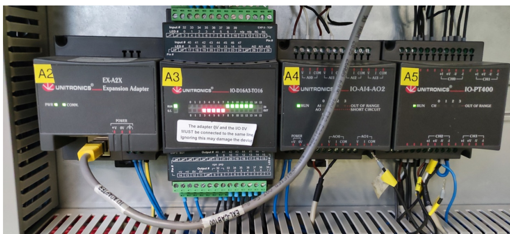
Slika 14. Ekspanzijski moduli PLC uređaja
