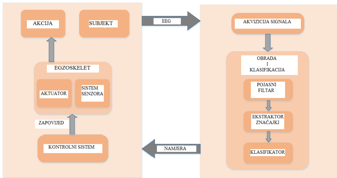
Slika 11. Komponente sistema [10]
