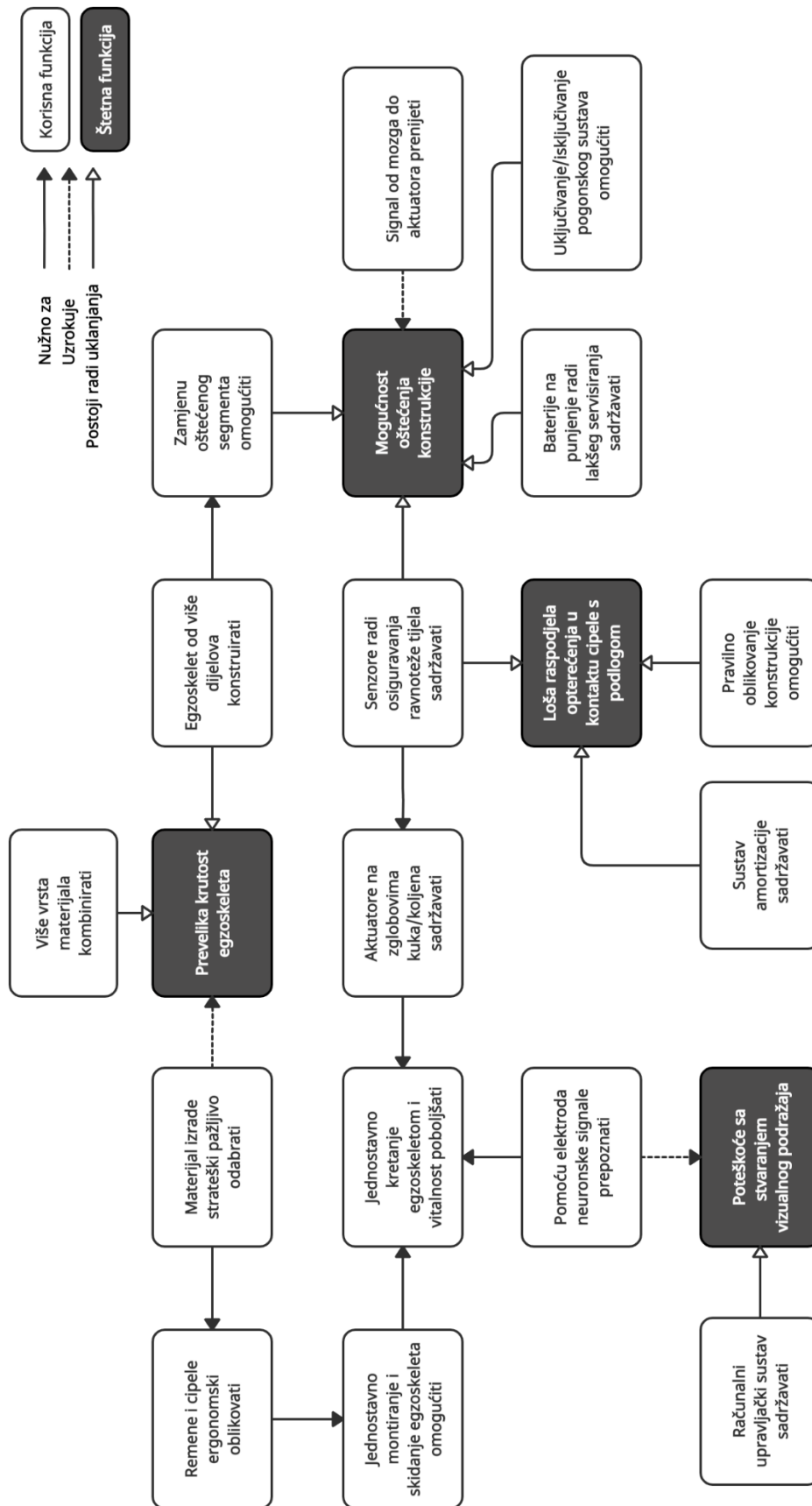
Slika 25. Model relacija
