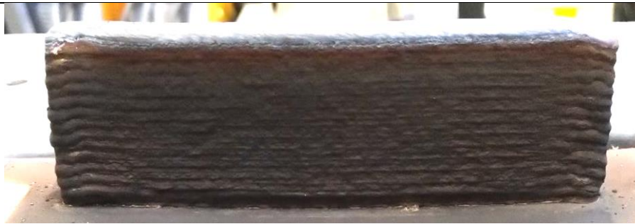
Slika 24. Navareni zid dupleks čelika
