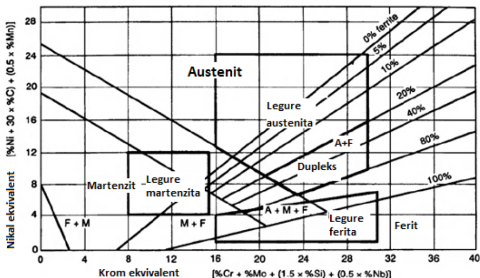
Slika 5. Schaefflerov dijagram [6]
