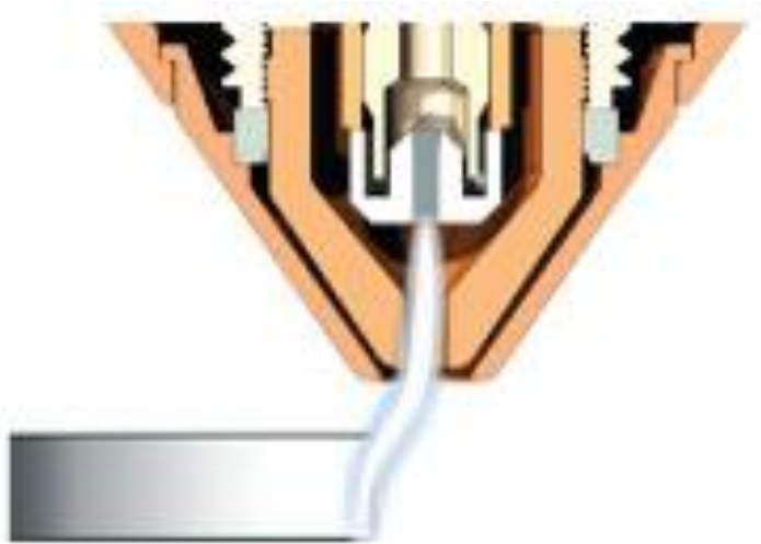
Slika 10. Povlačenje plazmenog luka [3]
