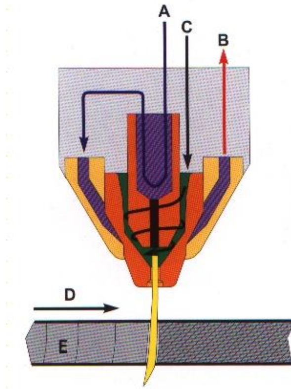
Slika 3. Suho plazma rezanje bez sekundarnog plina [2] (a) dovod vode, b) odvod vode, c) plazmeni plin, d) smjer rezanja, e) rub reza)
