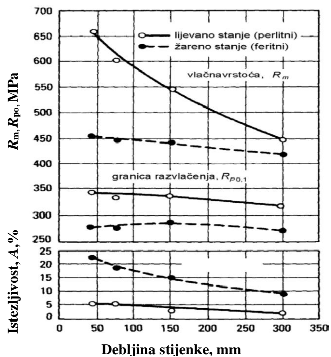
Slika 17: Utjecaj debljine stijenke na mehanička svojstva nodularnog lijeva [16]
