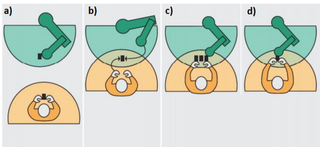
Slika 5. Različiti načini suradnje između čovjeka i robota prilikom montaže [10]
