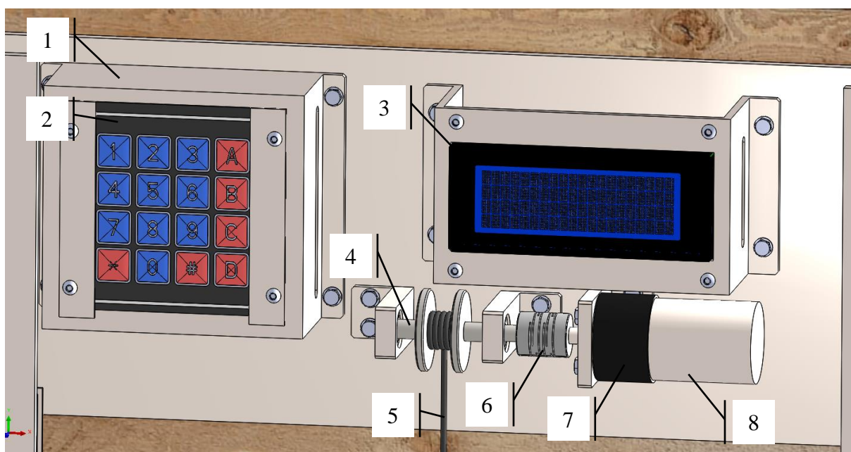
Slika 7. Unutrašnjost uređaja
