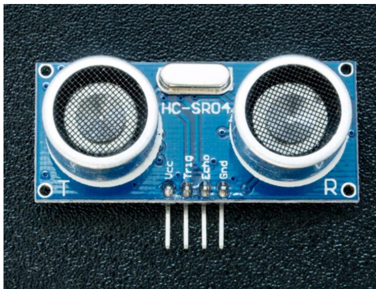
Slika 12. Ultrazvučni modul HC-SR04
