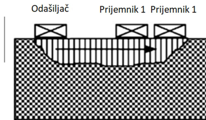
Slika 37. Površinsko ultrazvučno mjerenje [15]
