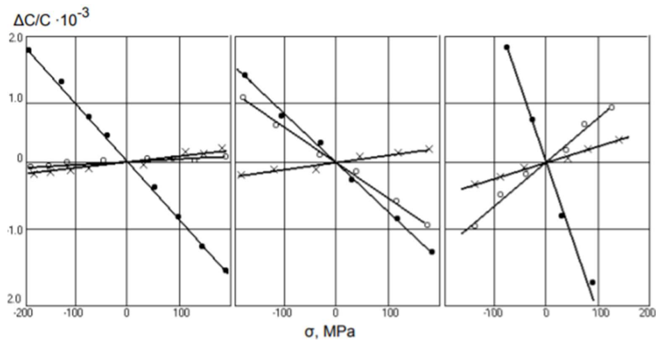
Slika 36. Utjecaj naprezanja na brzinu propagacije ultrazvučnih valova [15]
