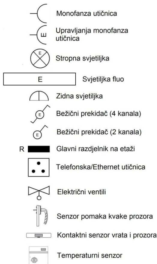
Slika 34. Simboli instalacija
