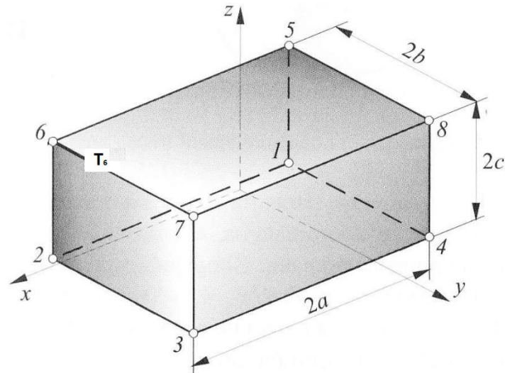
Slika 5. Osnovni prizmatični element [1]
