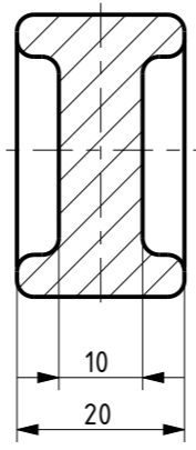
B-B 1:1
