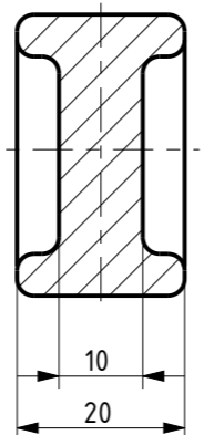
B-B 1:1
