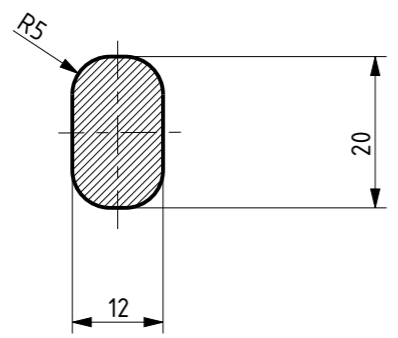
A-A 1:1
