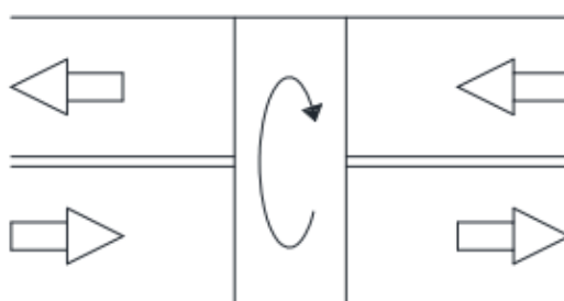
Slika 10 – Rotacijski regenerativni sustav [8]
