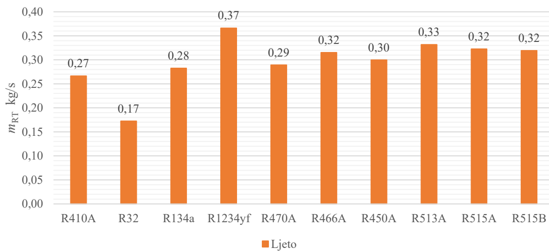
Slika 55 – Protoci radnih tvari za izmjereni proces
