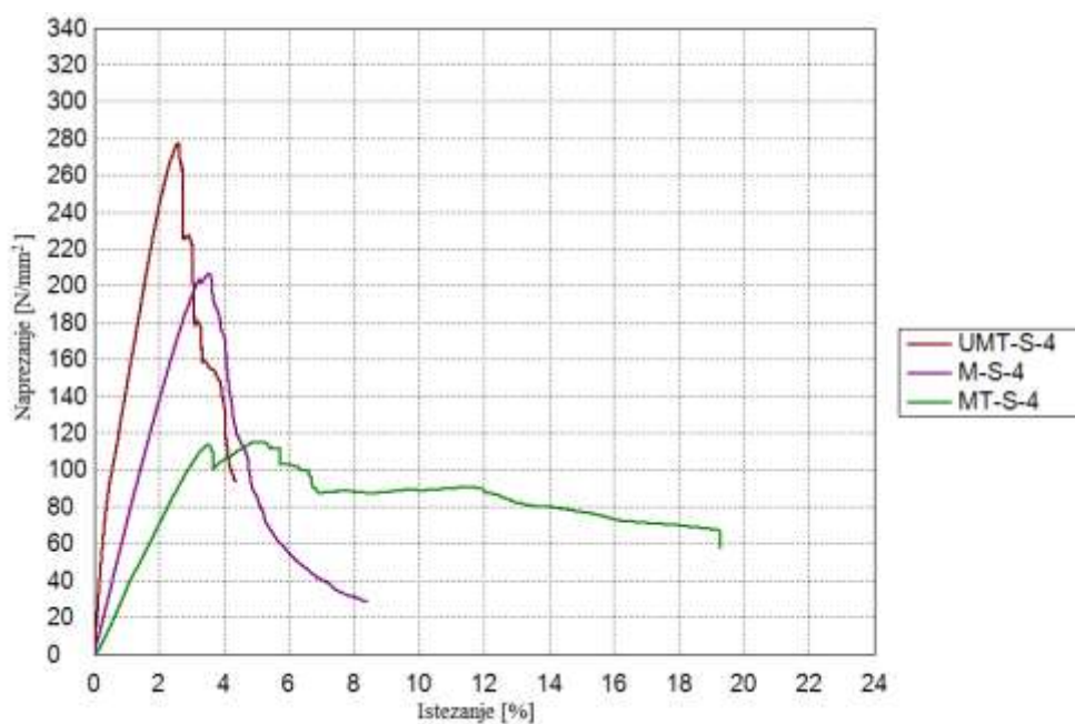
Slika 6.43. Dijagram savojnog naprezanja – istežanje usporedno za sve kompozite
