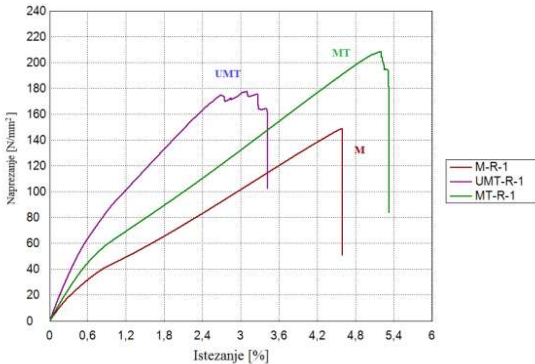
Slika 6.35. Dijagram rasteznog napreznosti-istežanja za sve ispitivane kompozite
