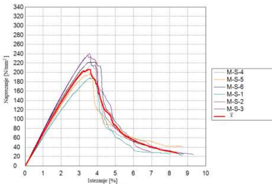
Slika 6.42. Dijagram savojnog naprezanja – istežanje za mat kompozit
