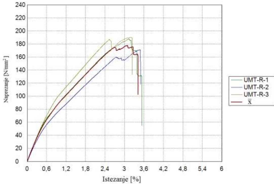
Slika 6.34 Dijagram rasteznog napreznosti-istežanja kompozita UMT-R
